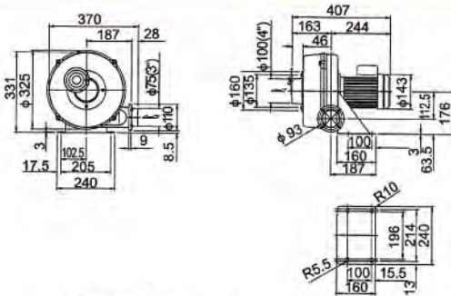
HTB75-032 2-stage
